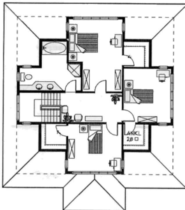
Grundrissplan Dachgeschoss
