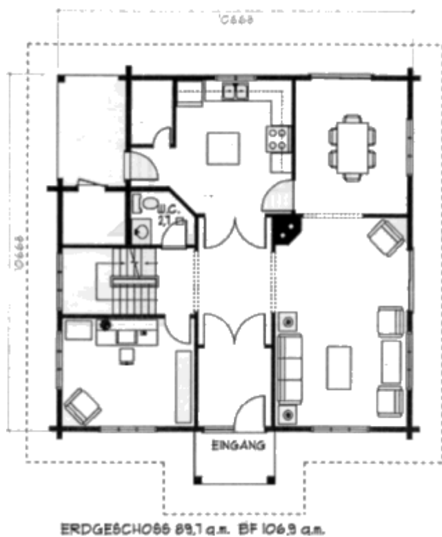
Grundrissplan Erdgeschoss
