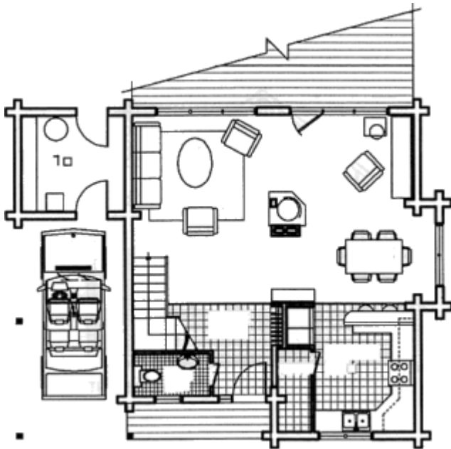
Grundrissplan Erdgeschoss
