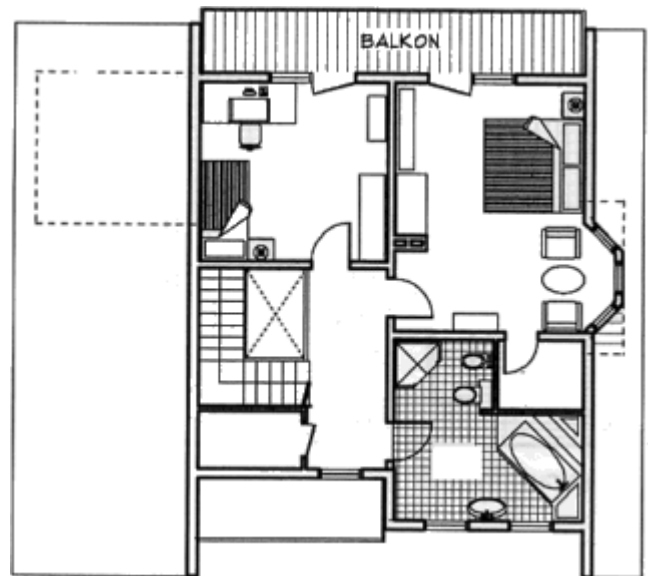
Grundrissplan Obergeschoss
