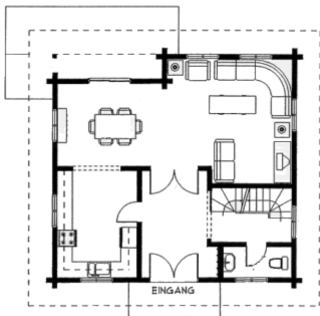
Grundrissplan Erdgeschoss
