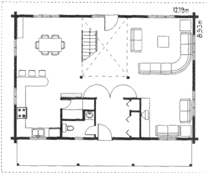
Grundrissplan Erdgeschoss
