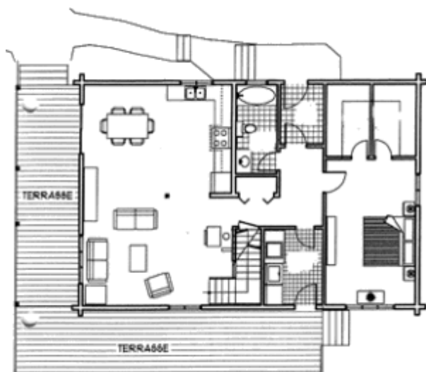
Grundrissplan Erdgeschoss
