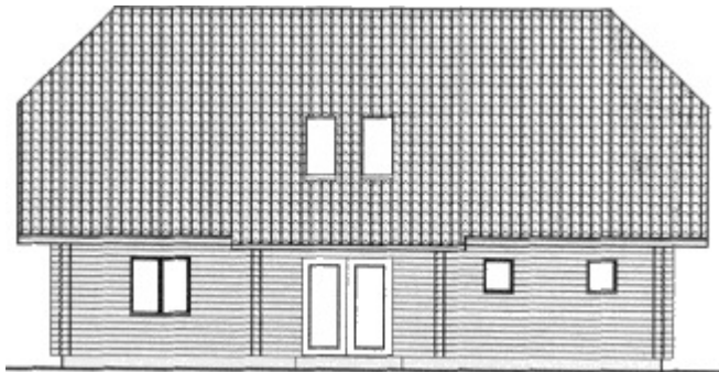
Frontansicht
