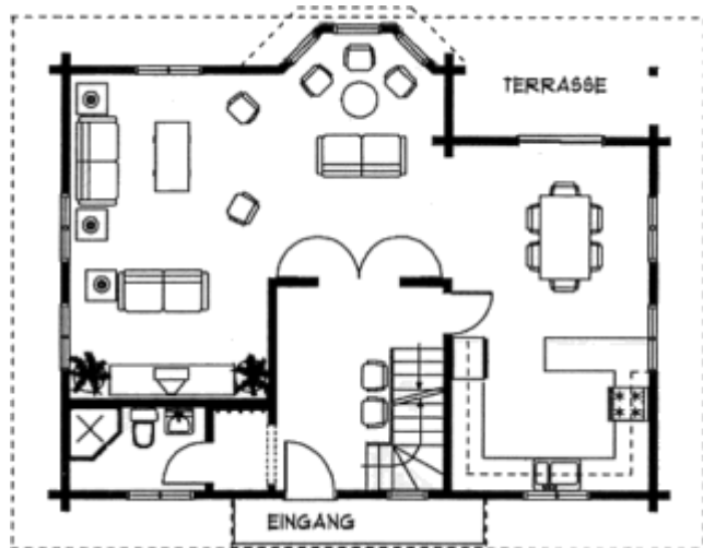
Grundrissplan Erdgeschoss
