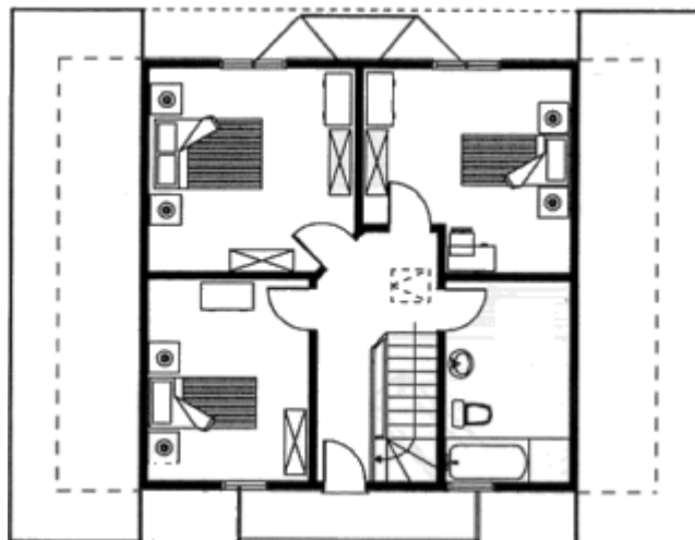
Grundrissplan Dachgeschoss
