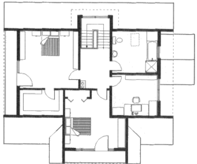
Grundrissplan Dachgeschoss
