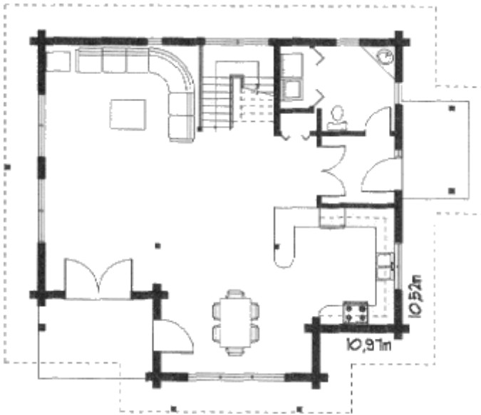
Grundrissplan Erdgeschoss
