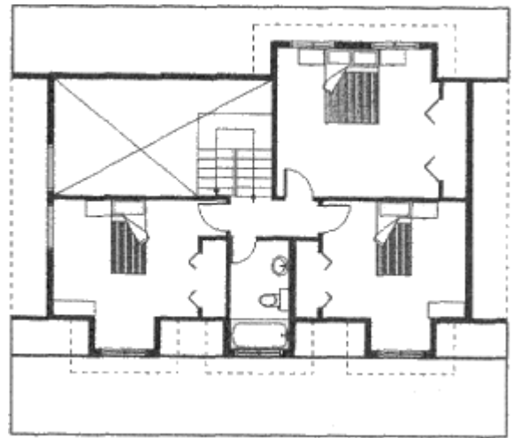
Grundrissplan Dachgeschoss
