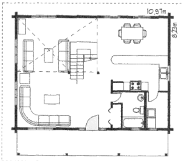
Grundrissplan Erdgeschoss
