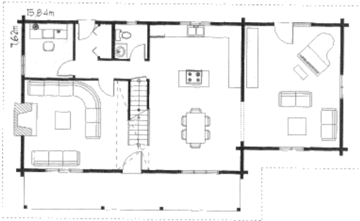
Grundrissplan Erdgeschoss
