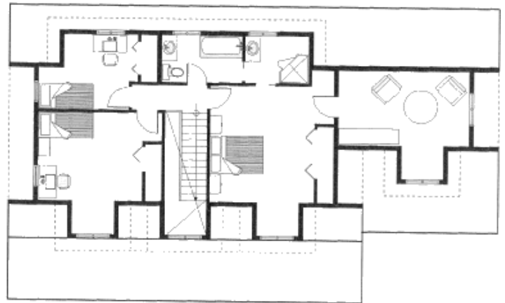
Grundrissplan Dachgeschoss
