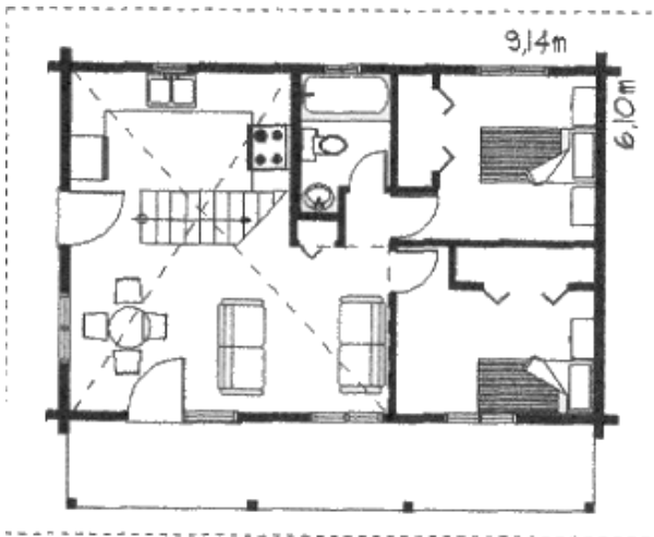
Grundrissplan Erdgeschoss
