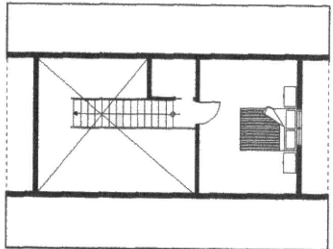
Grundrissplan Obergeschoss
