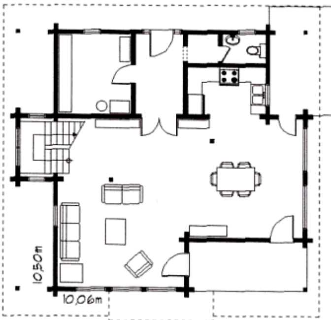
Grundrissplan Erdgeschoss
