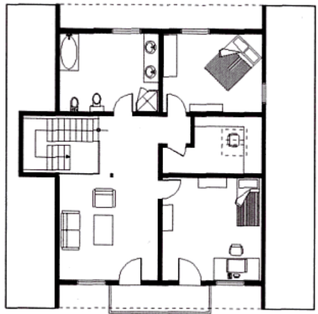
Grundrissplan Obergeschoss
